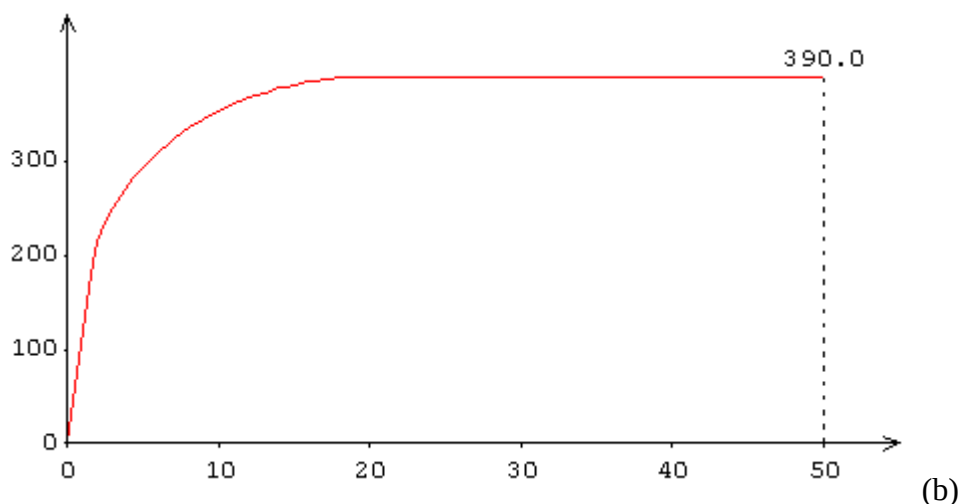
Рис.7. Диаграмма для арматуры согласно Eurocode 2 при 20 °C (а) и 500 °C (б)
