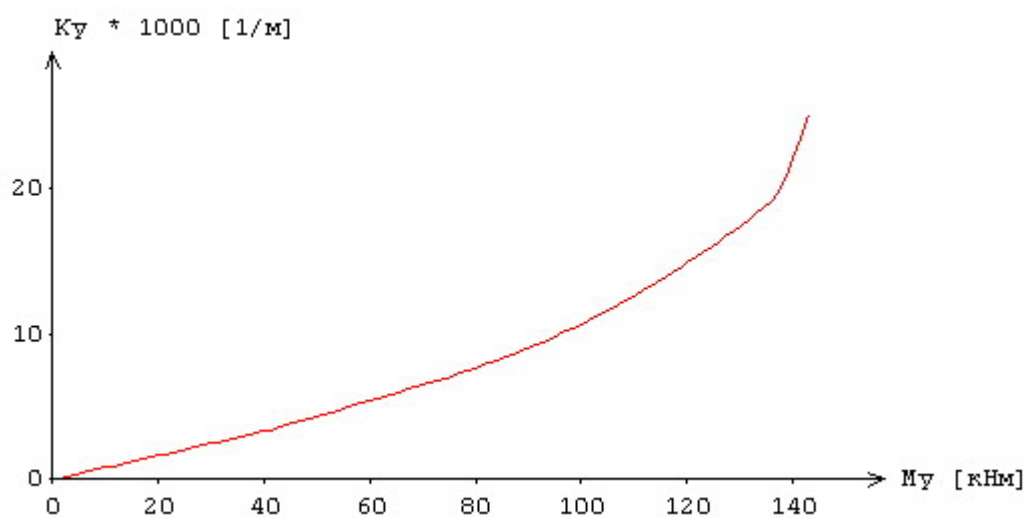
Рис.5. Зависимость «кривизна-момент» при N = 1200кН по [1]
