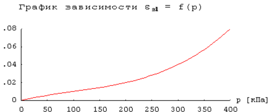
Рис.2. Пример зависимости относительной просадочности от давления
