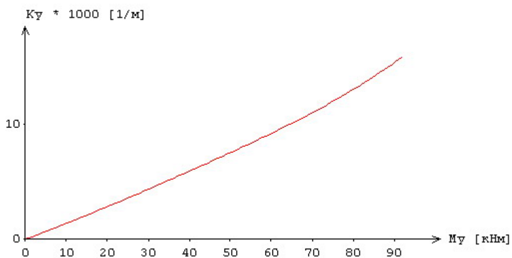
Рис.8. Зависимость «кривизна-момент» при N = 1200 \text{ кН} по [2]
