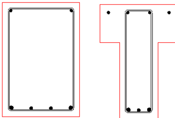
Рис.1. Виды сечений
