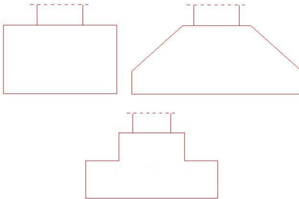
Рис.1 Сечения фундамента
