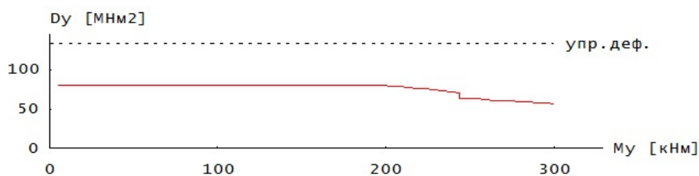
Рис. 13. Пример зависимости жесткости от момента для колонны
