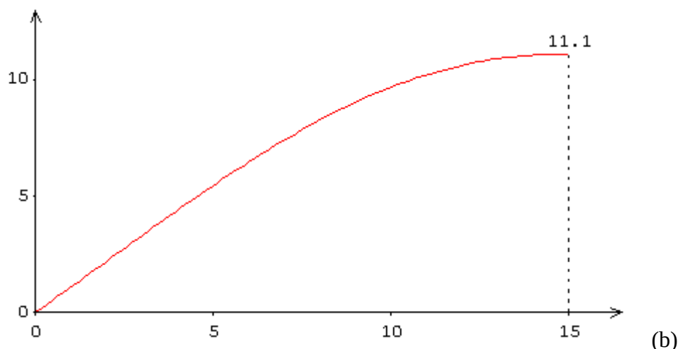
Рис.5. Диаграмма для сжатого бетона согласно Eurocode 2 при 20 °C (a) и 500 °C (b)
