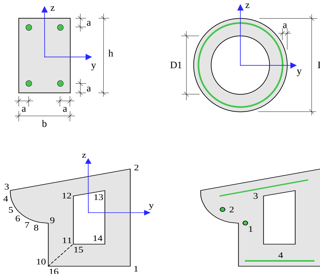
Рис. 2. Сечения
