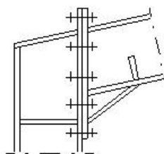
Рис. 2. Наклонный ригель
