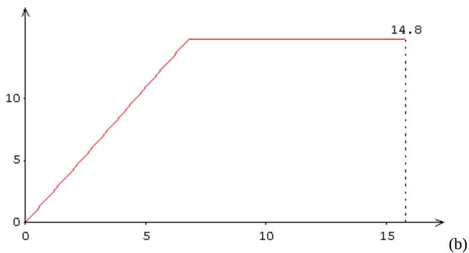
Рис.4. Диаграмма для сжатого бетона согласно СТО НИИЖБ при 20 °С (а) и 500 °С (б)
