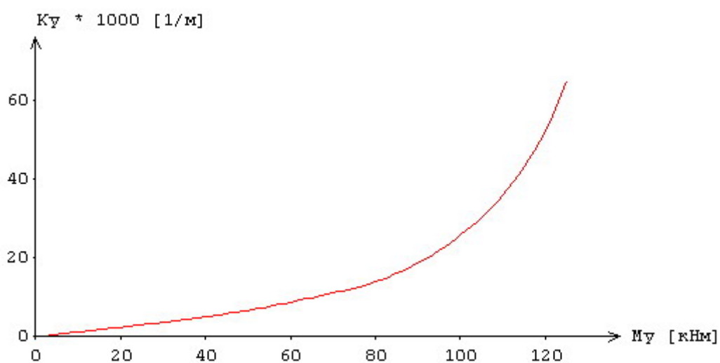
Рис.6. Зависимость «кривизна-момент» при N = 500кН по [2]
