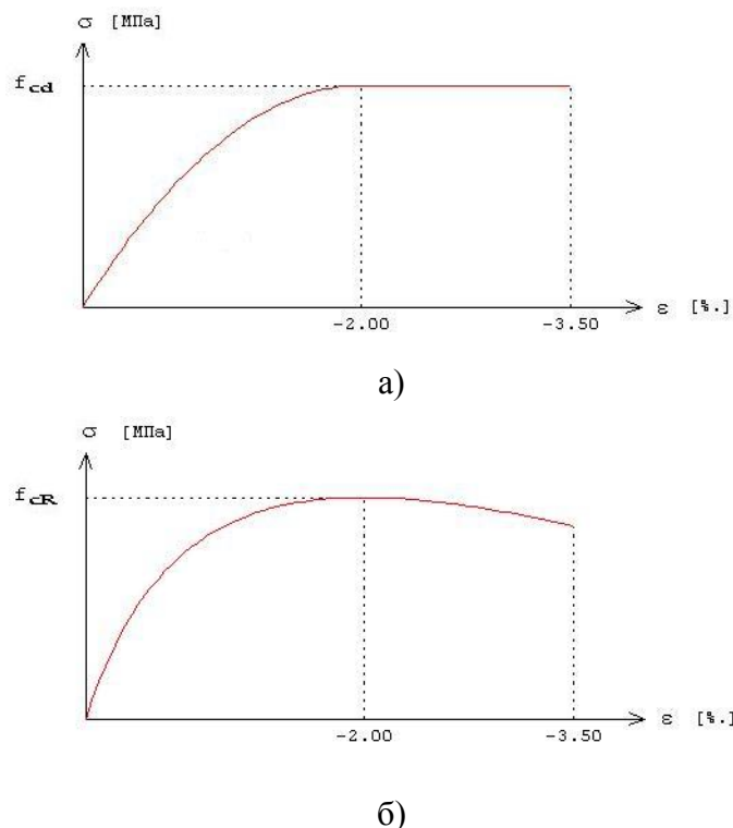
Рис. 4. Диаграммы деформирования сжатого бетона:
