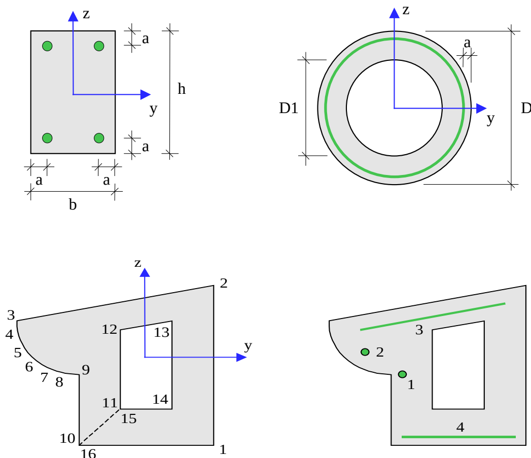
Рис. 4. Сечения
