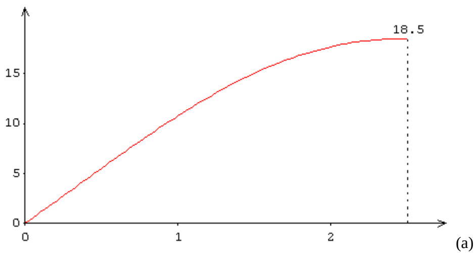
Рис.4. Диаграмма для сжатого бетона согласно СТО НИИЖБ при 20 °С (а) и 500 °С (б)
