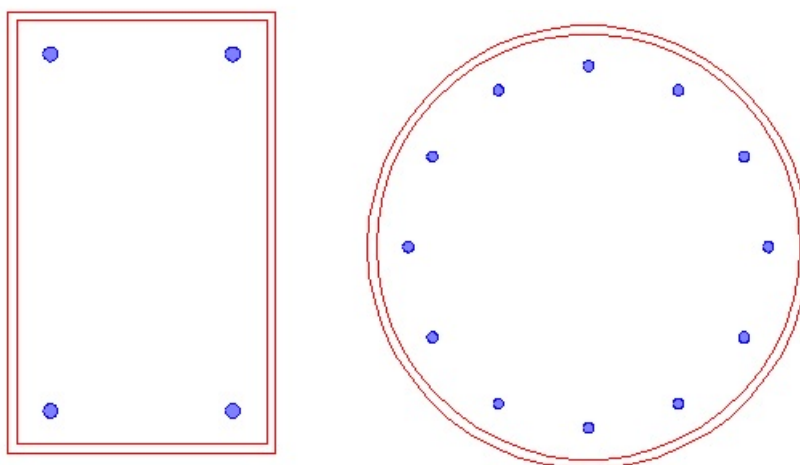
Рис. 7. Трубобетонные сечения
