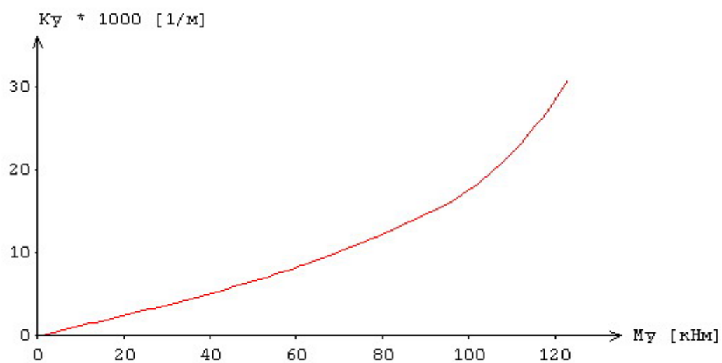
Рис.7. Зависимость «кривизна-момент» при N = 800 \text{ кН} по [2]
