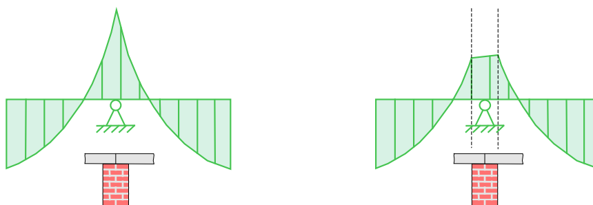
Рис. 7. Учёт ширины опирания при определении моментов
