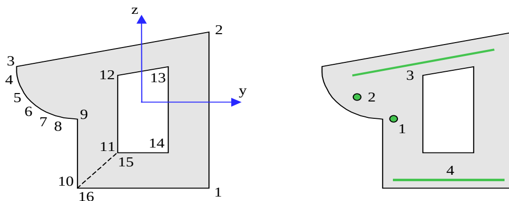
Рис. 4. Сечения
