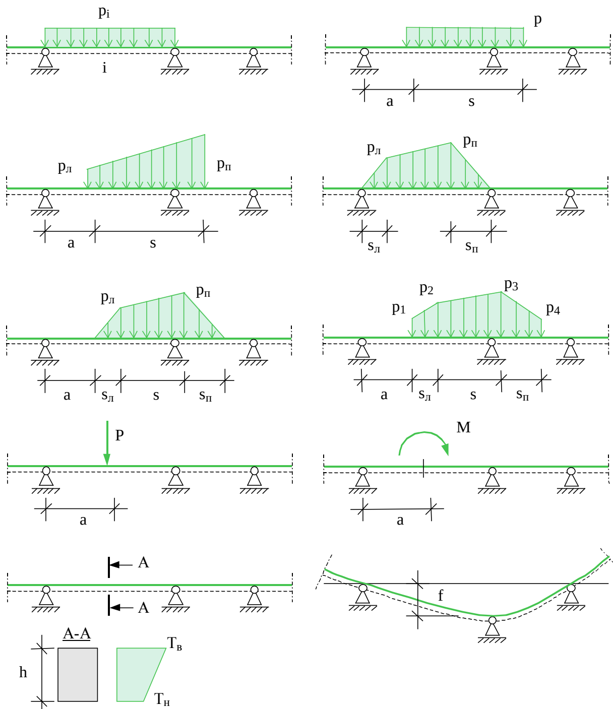
Рис.3. Виды нагрузок
