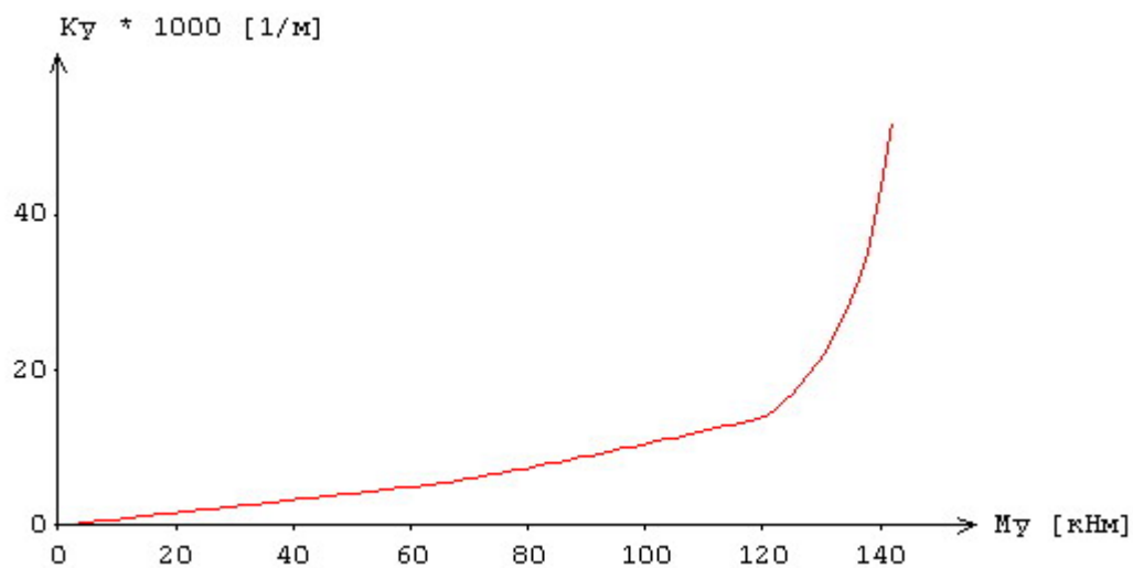
Рис.4. Зависимость «кривизна-момент» при N = 800кН по [1]
