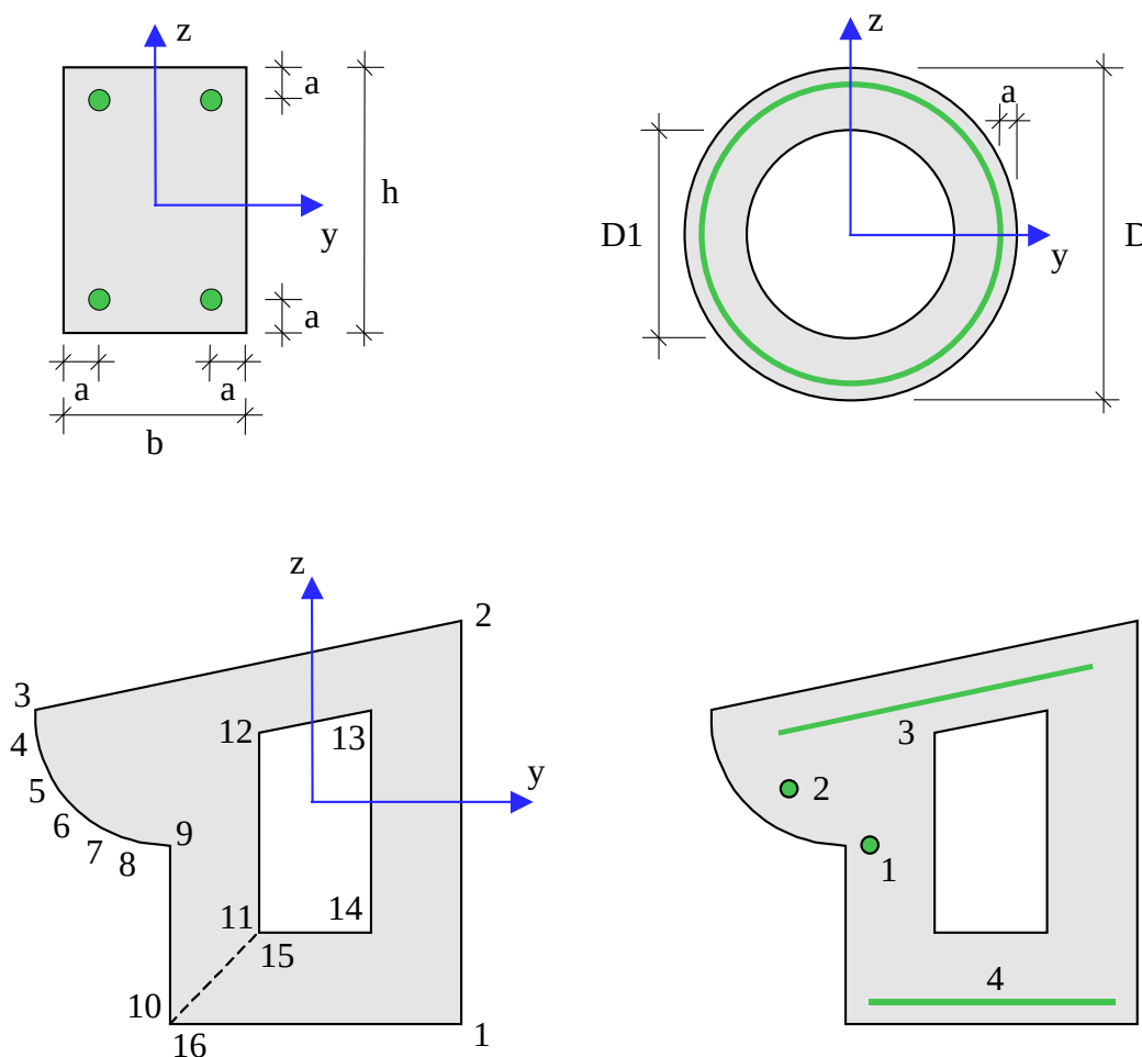
Рис. 1. Сечения
