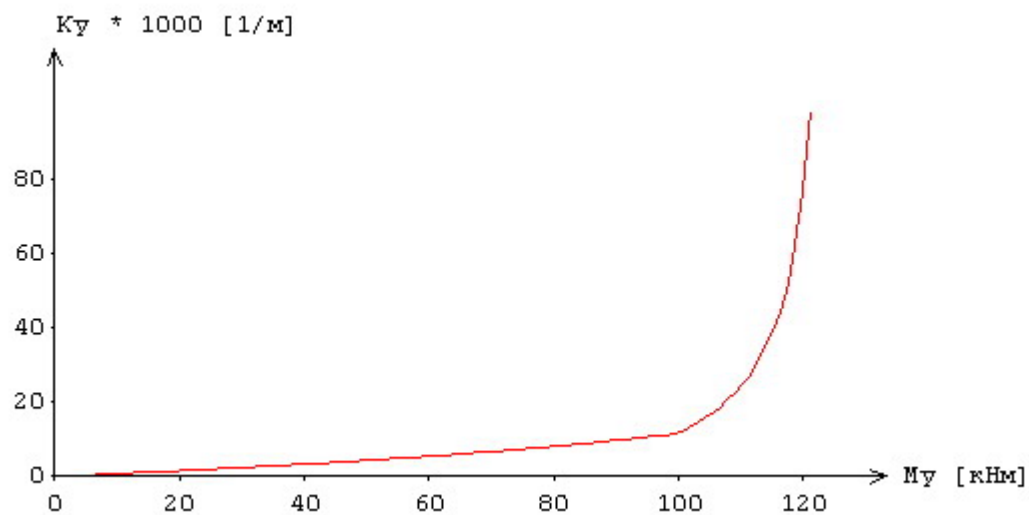
Рис.3. Зависимость «кривизна-момент» при N = 500кН по [1]
