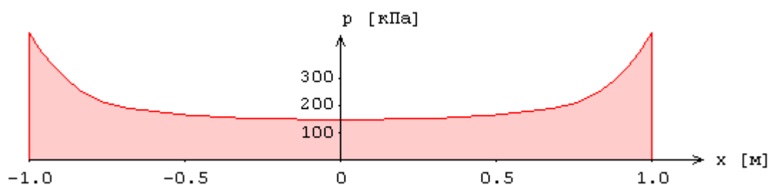
Рис.4. Пример распределения давления под подошвой абсолютно жесткого фундамента
