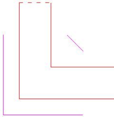
Рис.3. Расчетный контур при продавливании углом стены
