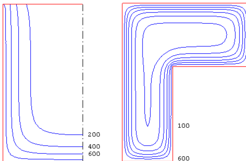
Рис.3. Изотермы
