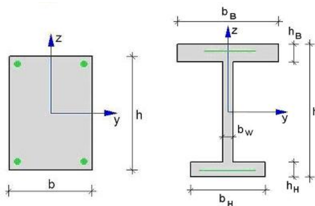
Рис. 1. Сечения
