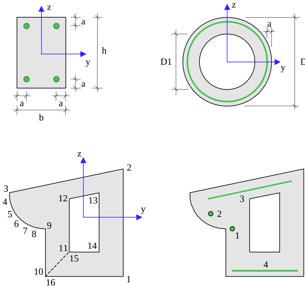
Рис. 1. Сечения
