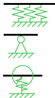
Рис. 5. Возможные условия закрепления плит
