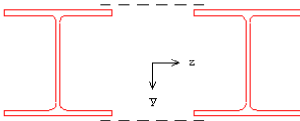
Рис. 5. Сечения сквозной колонны
